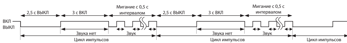
*3. Мигание светодиода при неисправности наружного блока
