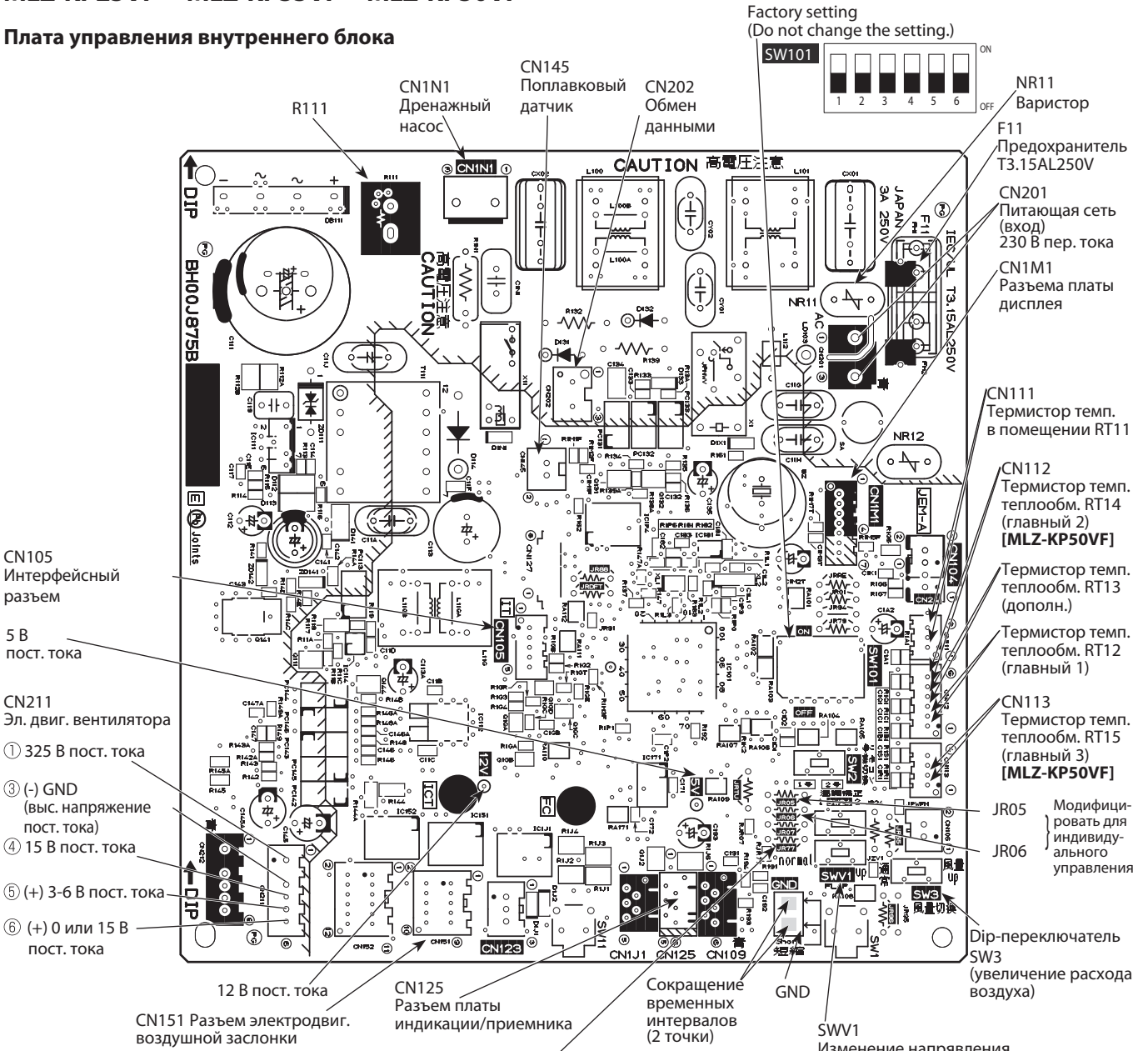
Термистор теплообменника [RT12, RT14, RT15 (главн.), RT13 (доп.)] Термистор темп. в помещении (RT11)
