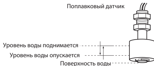
Поплавковый датчик
