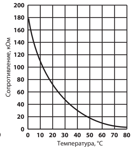
Термистор температуры теплоотвода (RT64)
