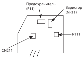
Плата управления внутреннего блока
