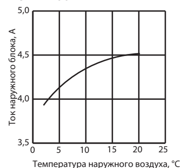
MUZ-HR60VF
