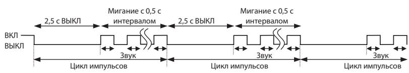
*3. Мигание светодиода при неисправности наружного блока
