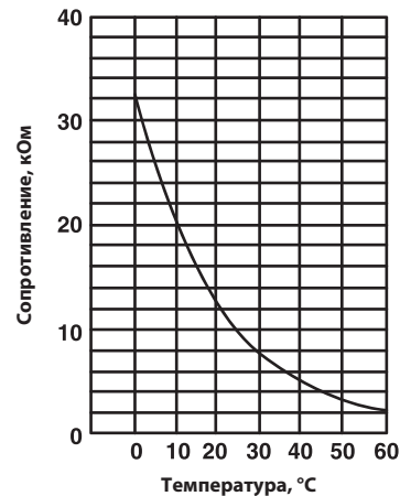
Термистор теплообменника внутреннего блока (RT12, RT14, RT15 (Глав.), RT13 (Вспом.)) Термистор температуры в помещении (RT11)
