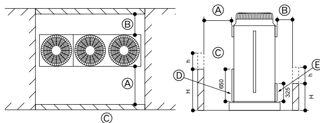
<Вид сбоку>
