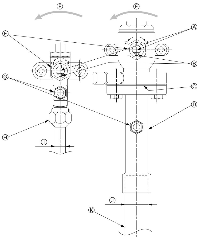
(На этой иллюстрации клапан показан в полностью открытом состоянии.)
