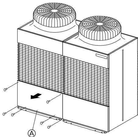
А Сервисная панель
