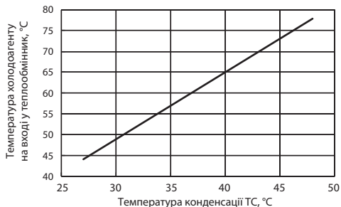
Мал. 2. Температура холодоагенту на вході в теплообмінник
