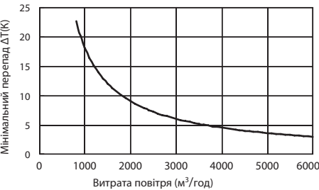
Мал. 3. Мінімальний перепад температури (режим нагрівання)
