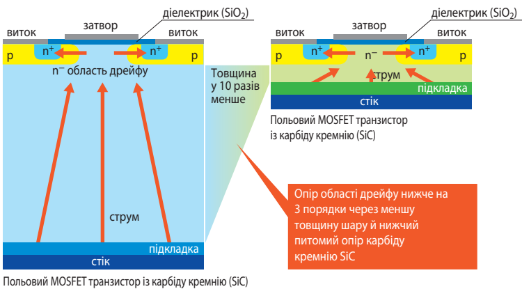
Спрощена структура польового транзистора MOSFET
