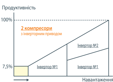
Одномодульний агрегат
