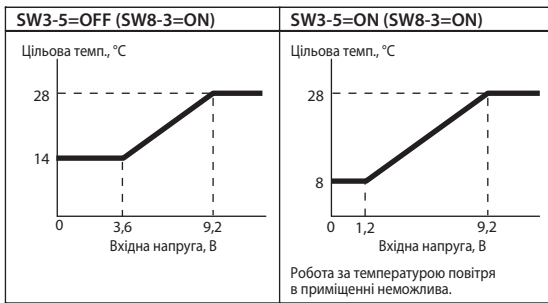
Мал. 4. Залежність цільової температури від керуючого сигналу
