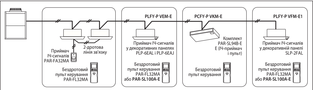
Приклад використання бездротових пультів
