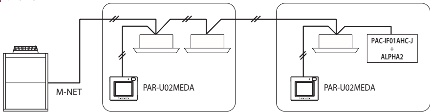
Пульт PAR-U02MEDA підключається у будь-яку точку сигнальної лінії M-NET без дотримання полярності. Групи формуються програмно.
