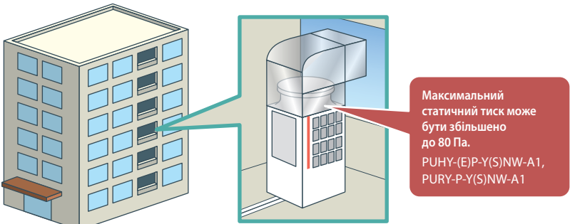
Групове встановлення на покрівлі поблизу огорожень або при щільній забудові
