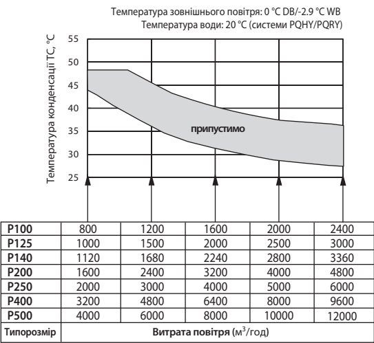
Мал. 1. Визначення припустимих значень температури конденсації
