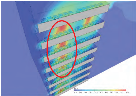
Поперехове встановлення у висотному будинку
